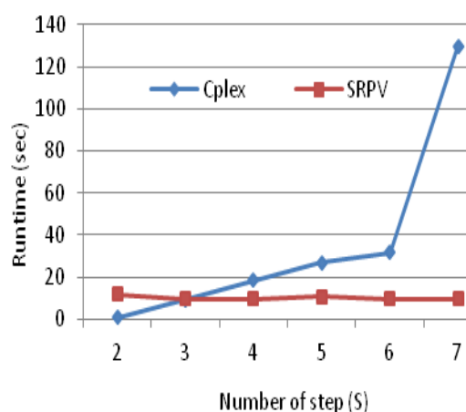
شکل 5: تغییر زمان حل با افزایش پله‌های تابع هدف
